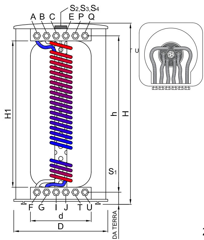
Schema tecnico SPAZIO PRO
