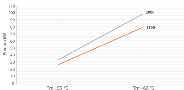
Potenza Scambiatore Superiore
