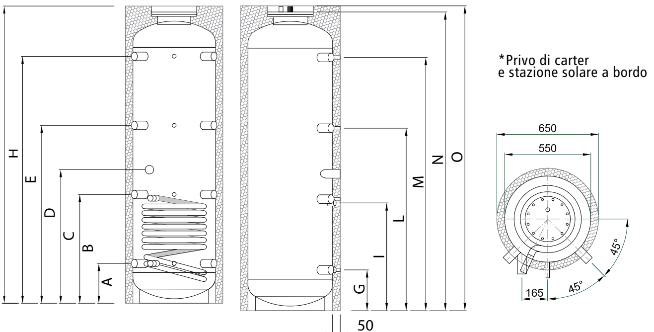
Schema tecnico ULTRAPR 401*
