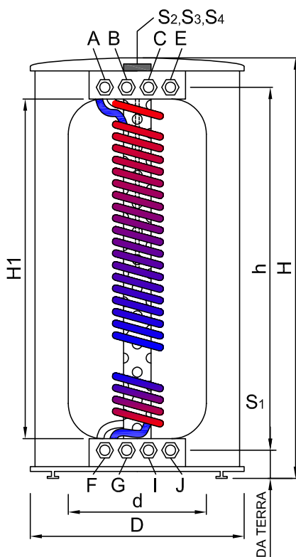
Schema tecnico SPAZIO
