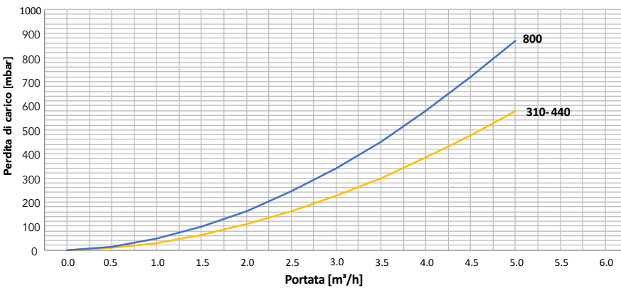
Perdite di carico scambiatore inferiore
