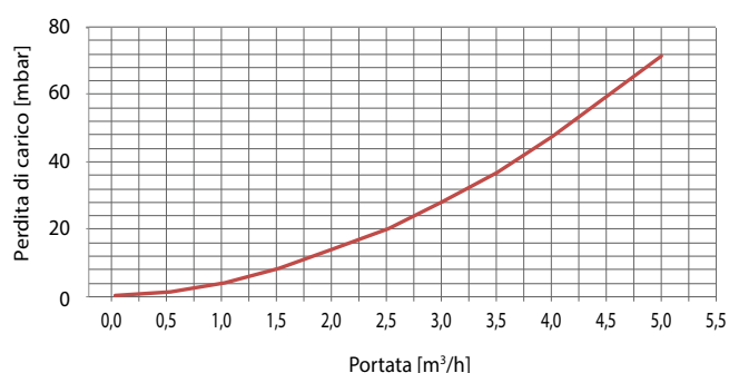
Perdite di carico scambiatore Solare ausiliario
