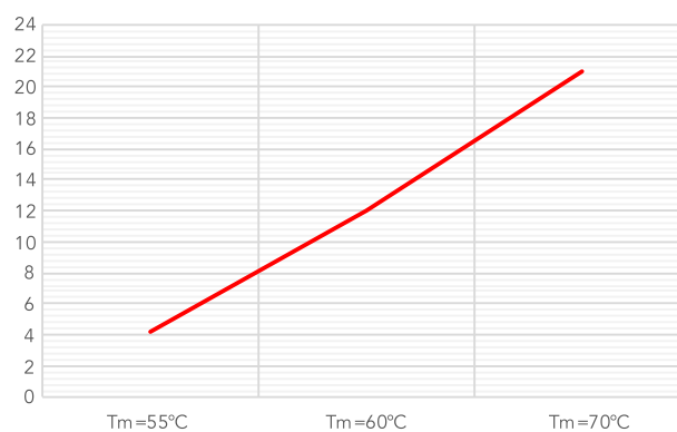
Potenza scambiatore Ausiliario
