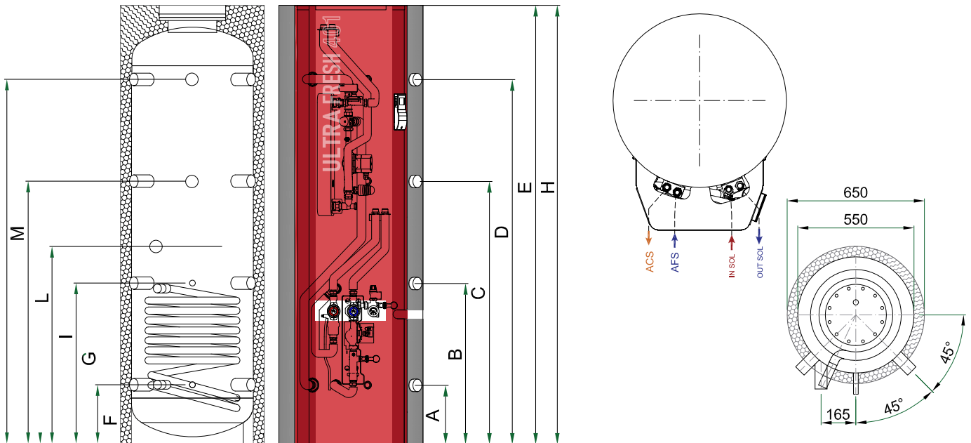
Schema tecnico ULTRAPR 401*
