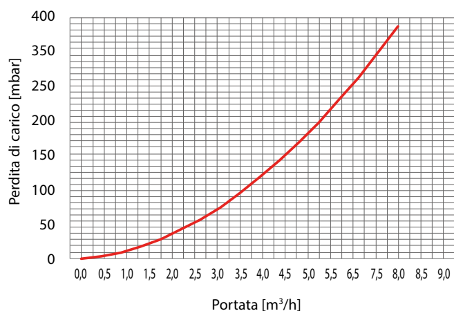
Perdite di carico scambiatore PDC
