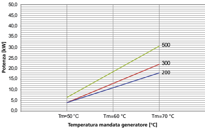
Perdite di Carico Scambiatore Superiore
