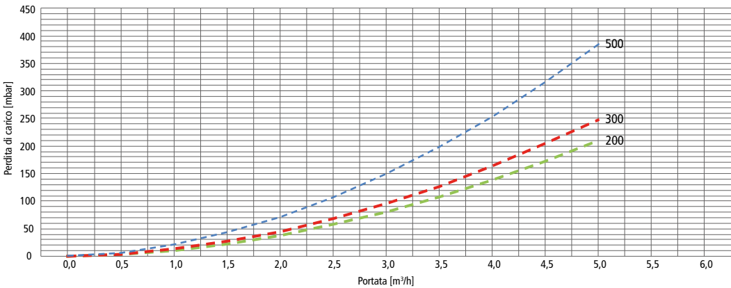
Perdite di Carico Scambiatore Inferiore
