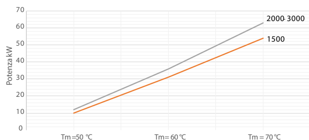
Potenza Scambiatore Superiore
