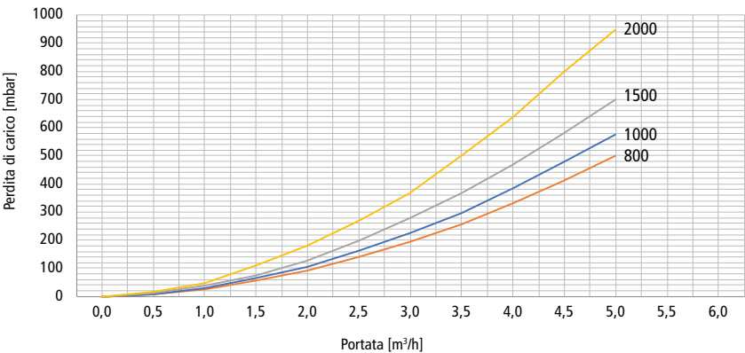
PERDITE DI CARICO SCAMBIATORE SUPERIORE
