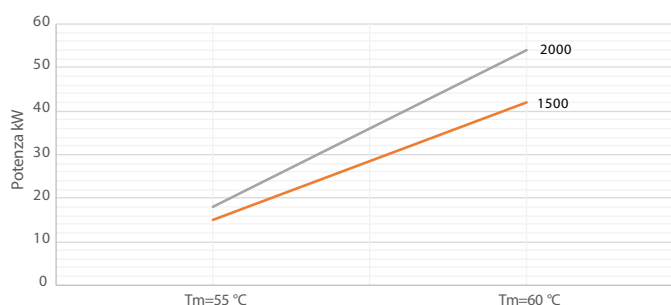
Potenza Scambiatore Inferiore
