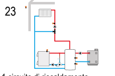
1 circuito di riscaldamento miscelato con caldaia a combustibile solido e riscaldamento integrativo (a richiesta)
