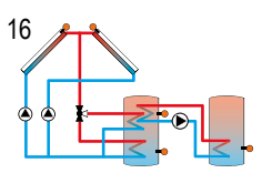
Sistema con collettori est/ovest e scambio termico
