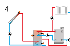
Sistema con 1 serbatoio, innalzamento temperatura ritorno e riscaldamento integrativo
