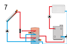
Sistema con 1 serbatoio stratificato e innalzamento temperatura ritorno
