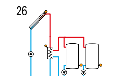
Impianto solare con 2 serbatoi, 1 scambiatore di calore esterno e comando pompa
