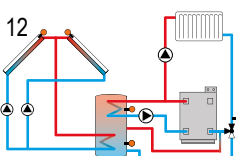
Sistema con collettori est/ovest, innalzamento temperatura ritorno e riscaldamento integrativo
