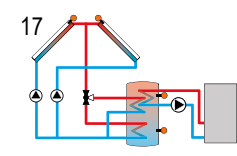
Sistema con collettori est/ovest e riscaldamento integrativo
