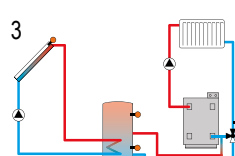
Sistema con 1 serbatoio e innalzamento temperatura ritorno
